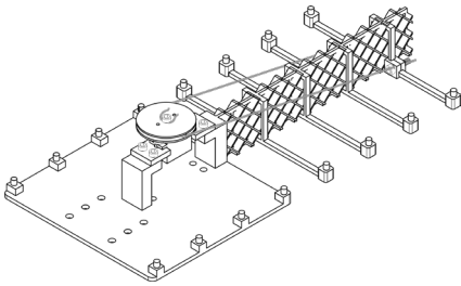
Steering Module
